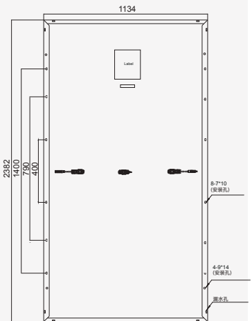
组件反面
