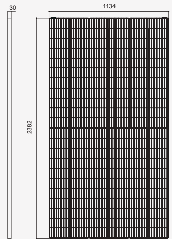
组件正面
