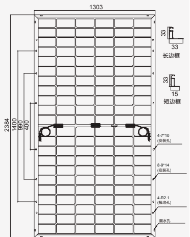
组件反面
