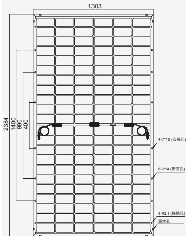
组件正面
