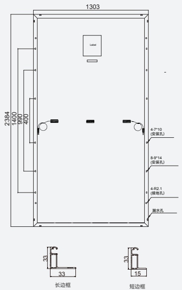
组件反面
