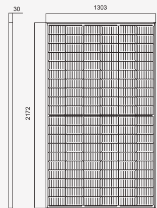
装配图(单位: mm)
