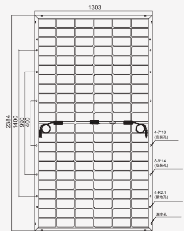
组件反面
