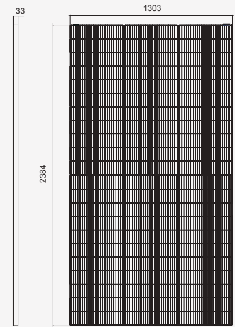
组件正面
