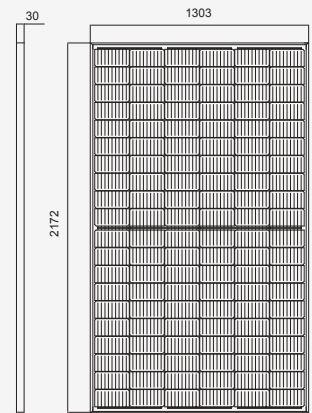
组件正面
