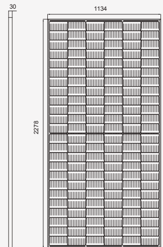
组件正面
