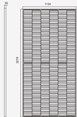
组件正面
