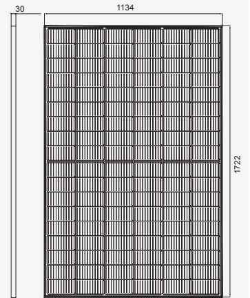
组件正面
