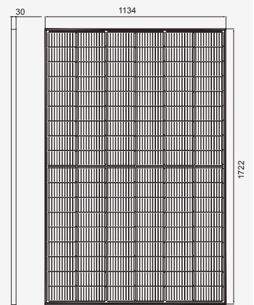
组件正面
