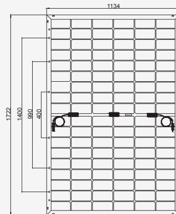
组件正面
