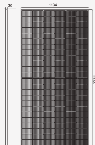
组件正面
