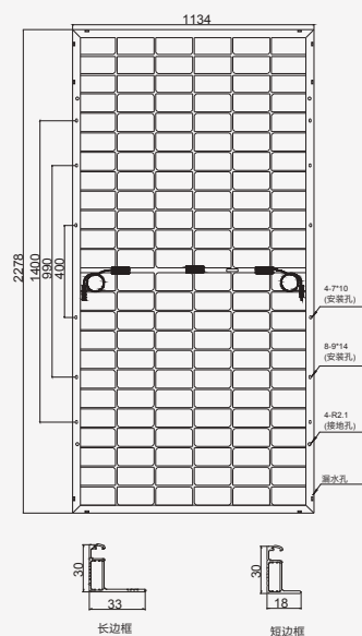
组件反面
