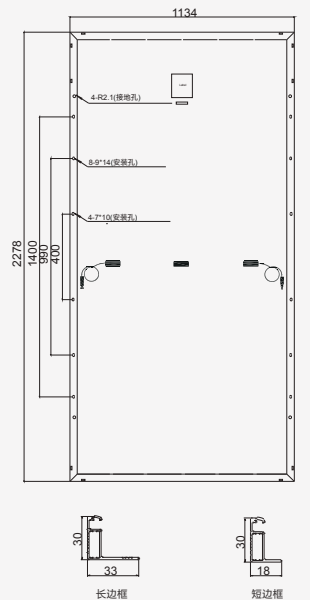
组件反面
