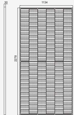
组件正面
