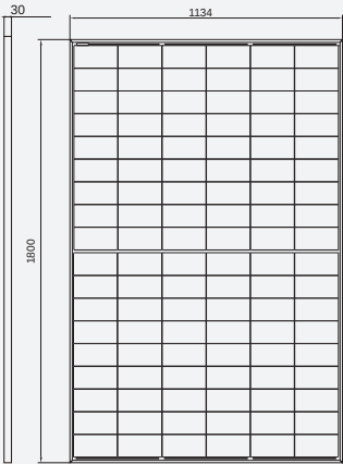
组件正面
