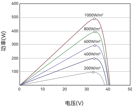
P-V曲线 (490W)
